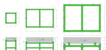
形状 I Shape I 形状 II Shape II 形状 III (レベルングブロック付) Shape III (With a leveling block)
